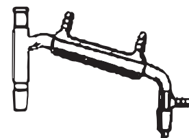
TENSIL-1602
